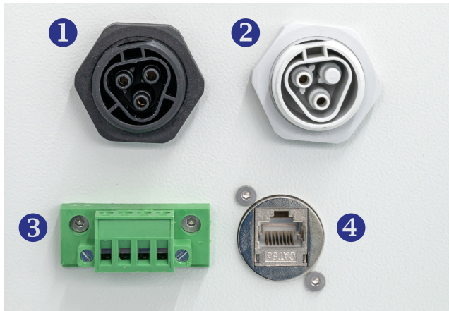
Außenansicht, Anschlüsse des Speichers
