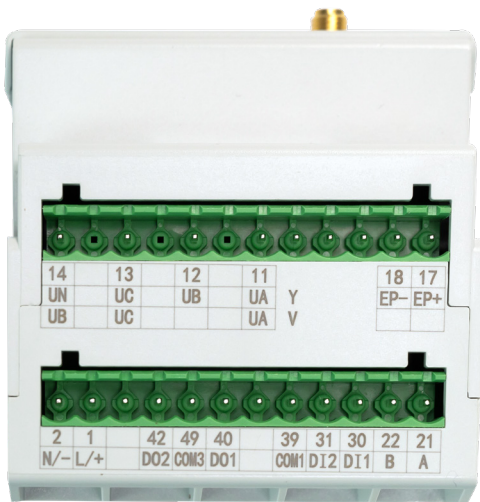
ADW220: Ansicht von oben
